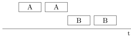
Abbildung 4.21: Der endliche Automat des temporalen Musters A meets B bleibt nach akzeptieren des ersten A stecken.
