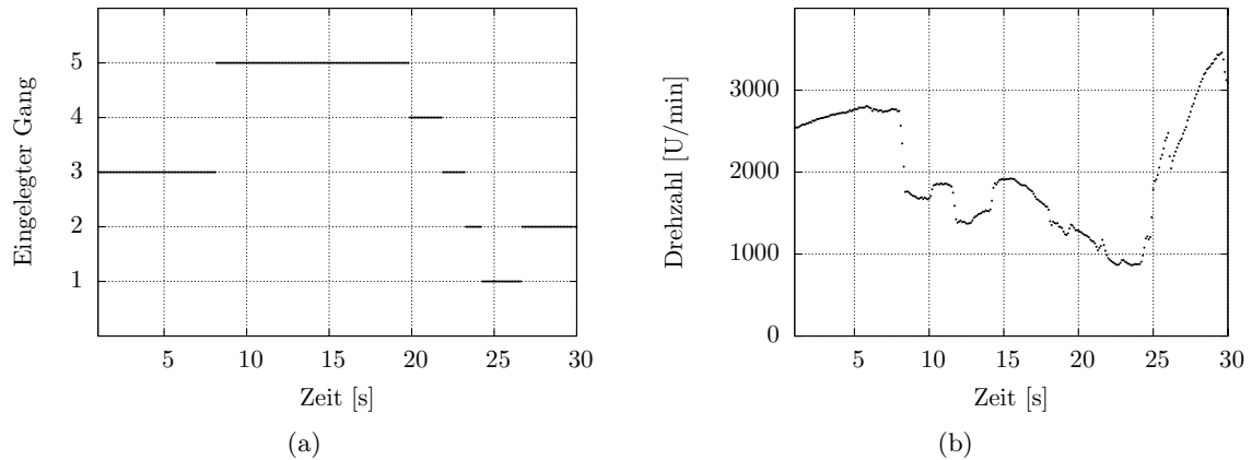
Abbildung 7.4: Beispiele für zwei aufgezeichnete Signale: (a) das diskrete Signal des eingelegten Gangs und (b) das kontinuierliche Signal für die gegenwärtige Motordrehzahl.
