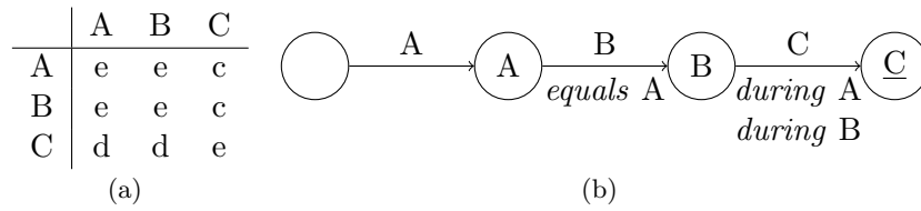
Abbildung 4.20: (a) ein temporales Muster (b) sein endlicher Automat
