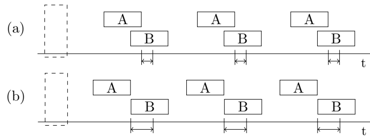
Abbildung 4.12: Obwohl die temporalen Muster A overlaps B und A meets B in beiden Intervallsequenzen gleich oft Vorkommen, berechnet der temporale Support einen doppelt so hohen Support für das Muster A meets B .
