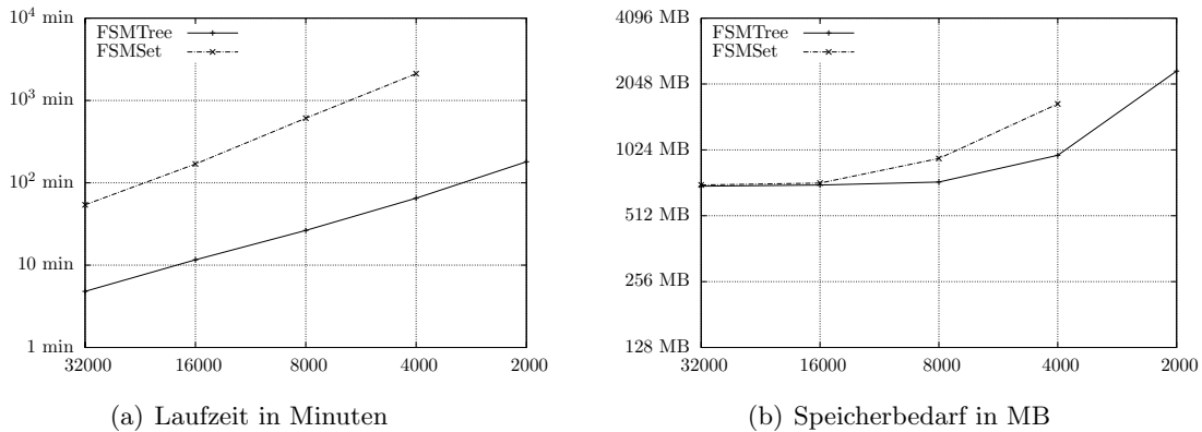
Abbildung 5.7: Effizienz der Verfahren auf CRM bei variierendem MinSup
